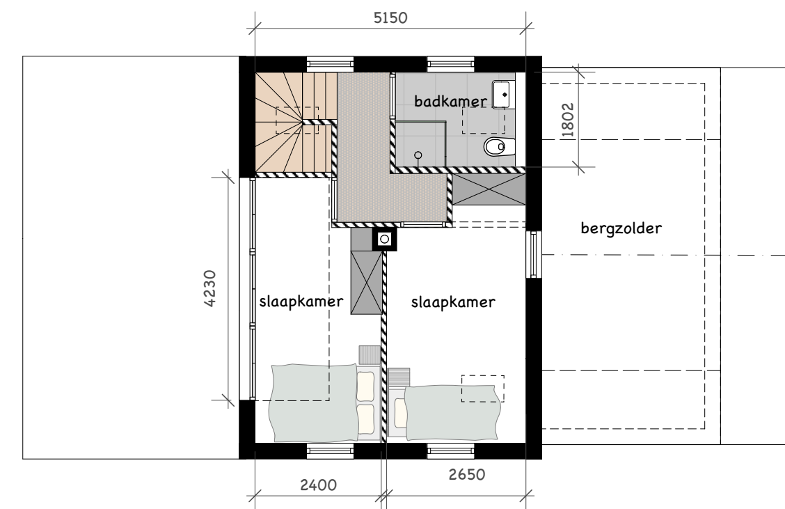
PLATTEGROND VERDIEPING
